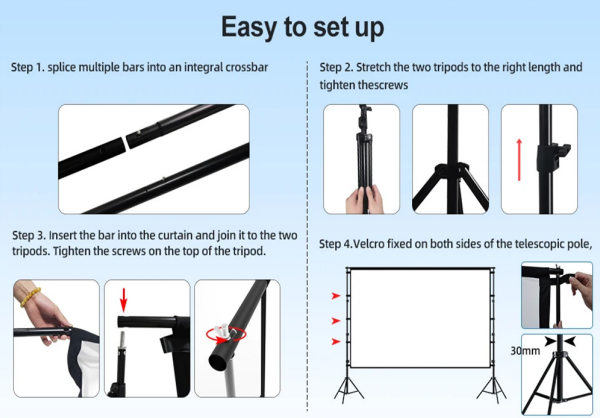
KHUNG MÀN KIỂU I-Shaped: OPS100W-T / OPS120W-T
